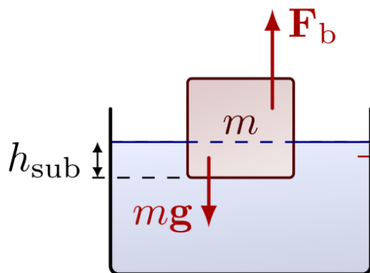
Figur 6.6: Oppdrift F_b , hvor oppdriftskraften beregnes ut fra volumet av væsken som fortrenses. Det fortrengte volumet er gitt som V_q = h_{\text{sub}} \cdot A , der h_{\text{sub}} er dybden av den nedsenkede delen av legemet, og A er arealet av bunnflaten.
